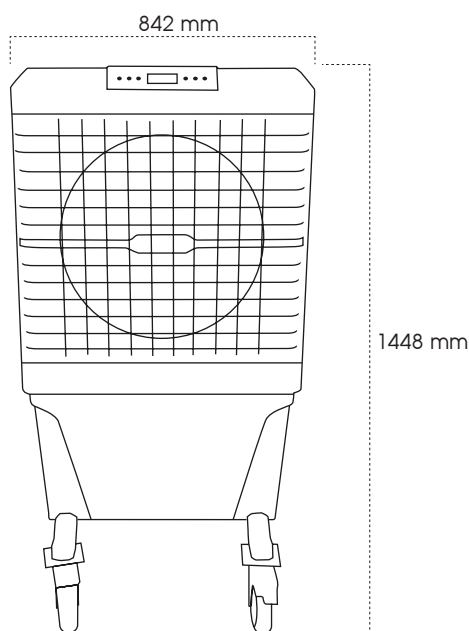
vista frontale
